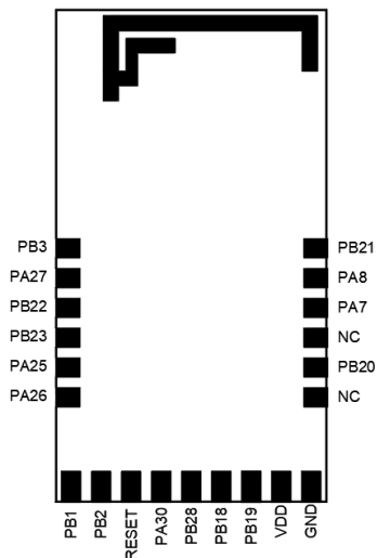
图 2 引脚分布
