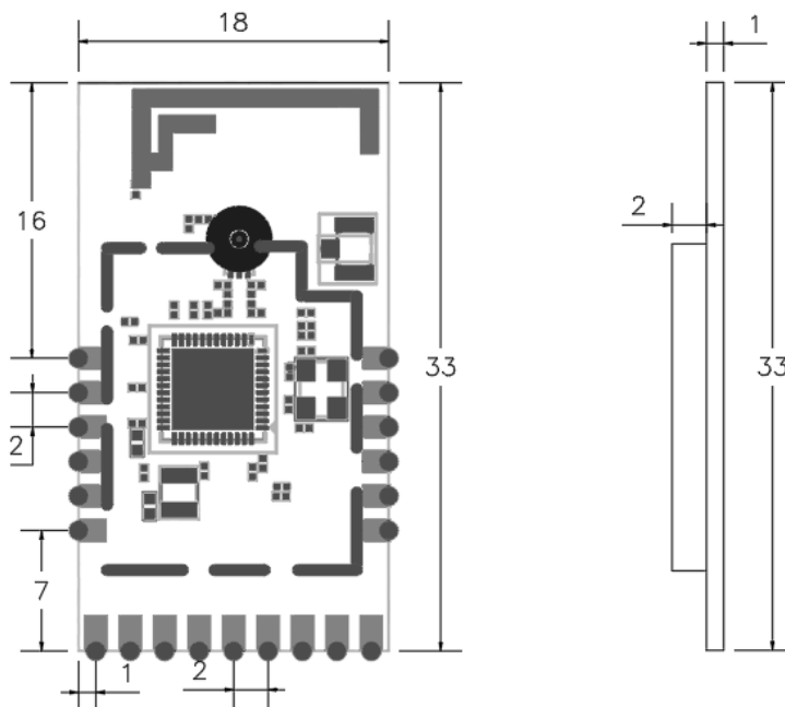
图 5 总装尺寸图 (单位: mm, 误差 \pm 0.1 , 外尺寸误差 \pm 0.2 )
