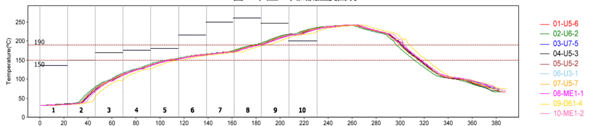
图 8 典型二次回流温度曲线
