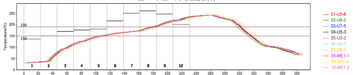
图 12 典型二次回流温度曲线
