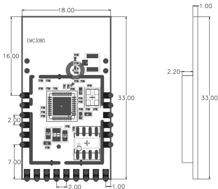
图 7 总装尺寸图 (单位: mm, 误差 \pm 0.1 , 外尺寸误差 \pm 0.2 )
